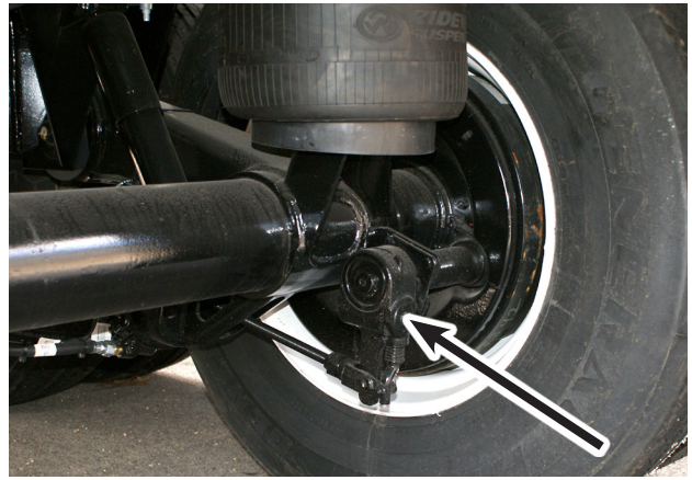
Slack Adjuster
